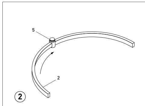
Переместите держатель (5) на середину трека
