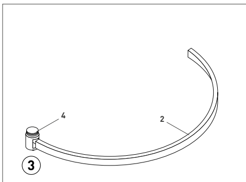
Установите на второй трек (2) держатель трека (4)
