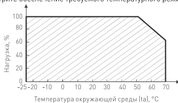
Рис. 3. Максимальная допустимая нагрузка, % от мощности источника
