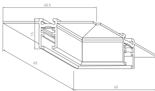
Коннектор угловой MAG-MICROCOSM-CON-FDW-L90-INT
