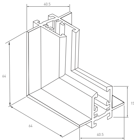
Коннектор угловой MAG-MICROCOSM-CON-FDW-L90
