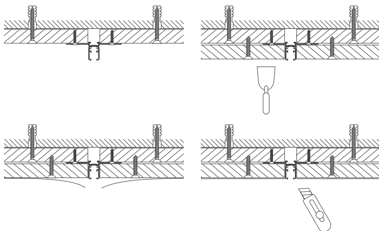
Рис. 3. Установка и подключение трека встраиваемым способом
