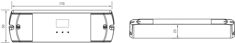
Рис. 1. Габаритный чертеж
