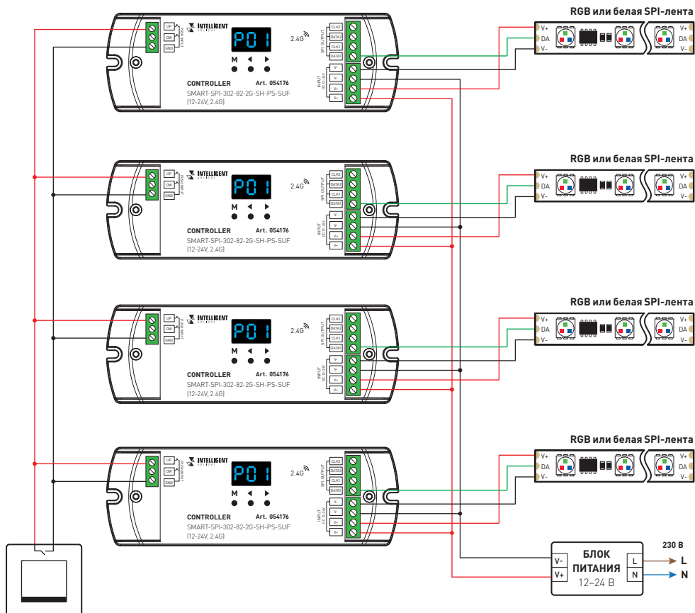
Рис. 3. Схема подключения нескольких контроллеров параллельно
