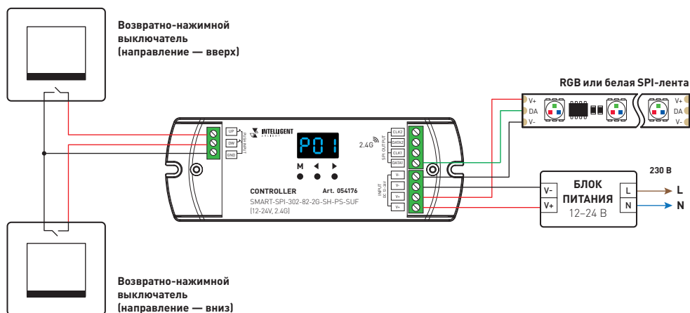
Рис. 2. Схема подключения контроллера при лестничном освещении
