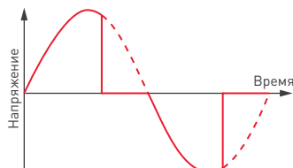
Диммирование с отсечкой заднего фронта. Используется для ламп накаливания и емкостной нагрузки, в том числе светодиодных источников света
