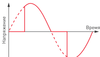
Диммирование с отсечкой переднего фронта. Используется для ламп накаливания и индуктивной нагрузки
