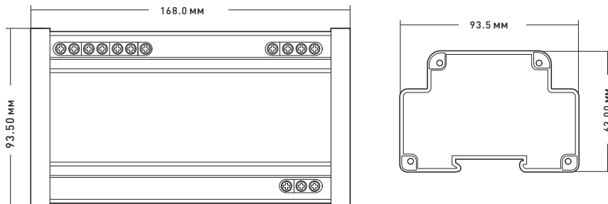
Рис. 1. Габаритный чертеж
