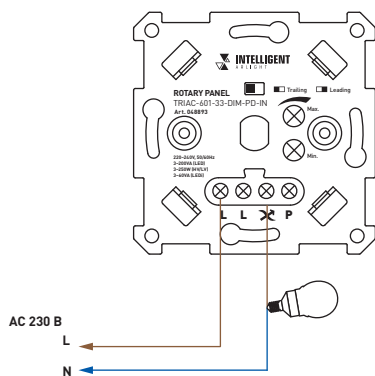
Рис. 2. Схема подключения панели TRIAC-601-33-DIM-PD-IN
