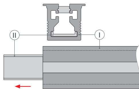
Рис. 1. Извлечение выдвижной пластины ② из профиля ①, вид сверху
