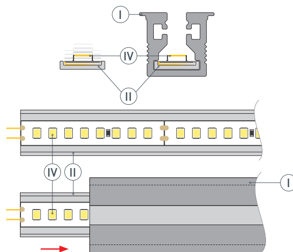
Рис. 2. Установка выдвижной пластины ② со светодиодной лентой ④ в профиль ①, вид сверху
