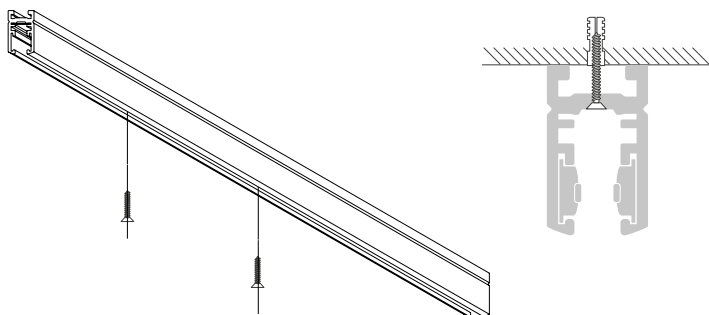
Рис. 4. Установка и подключение трека накладным способом
