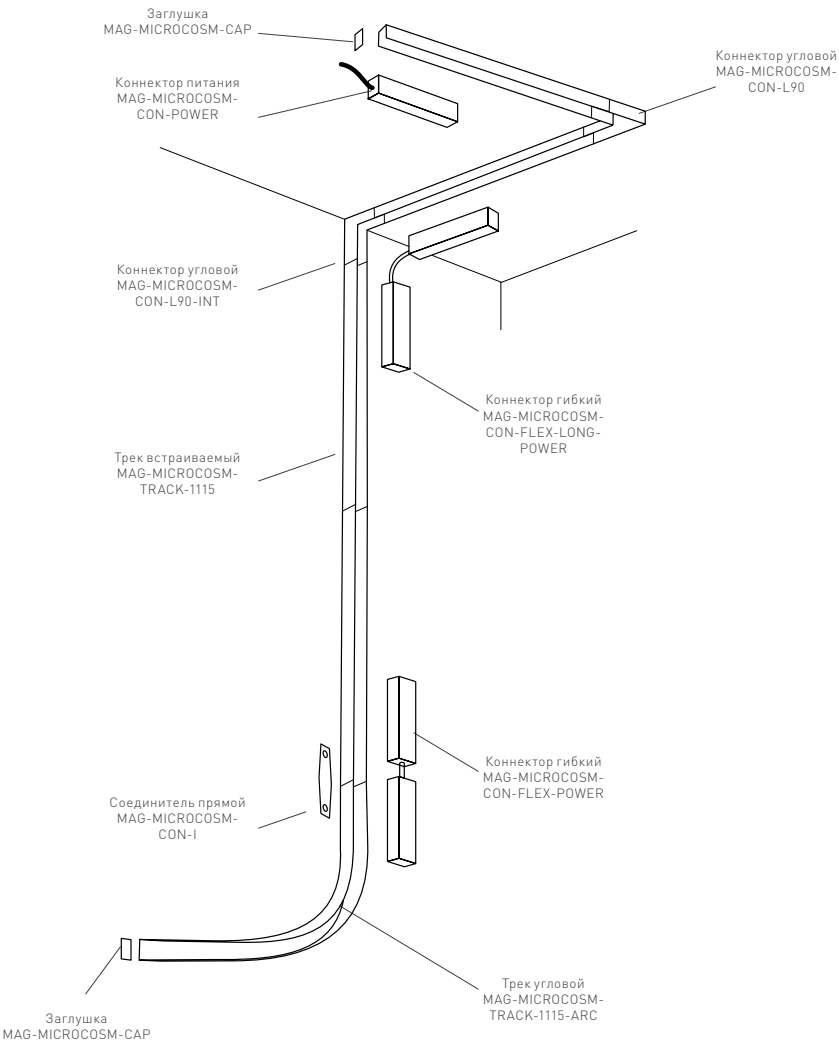
Рис. 3. Элементы и принцип построения разветвленной системы (накладной монтаж)
