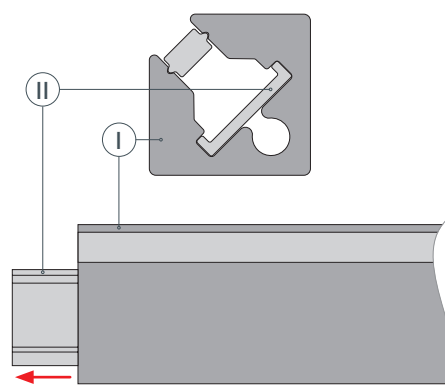
Рис. 1. Извлечение выдвижной пластины ② из профиля ①, вид сверху
