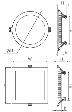
Рис. 1. Чертеж и габаритные размеры
