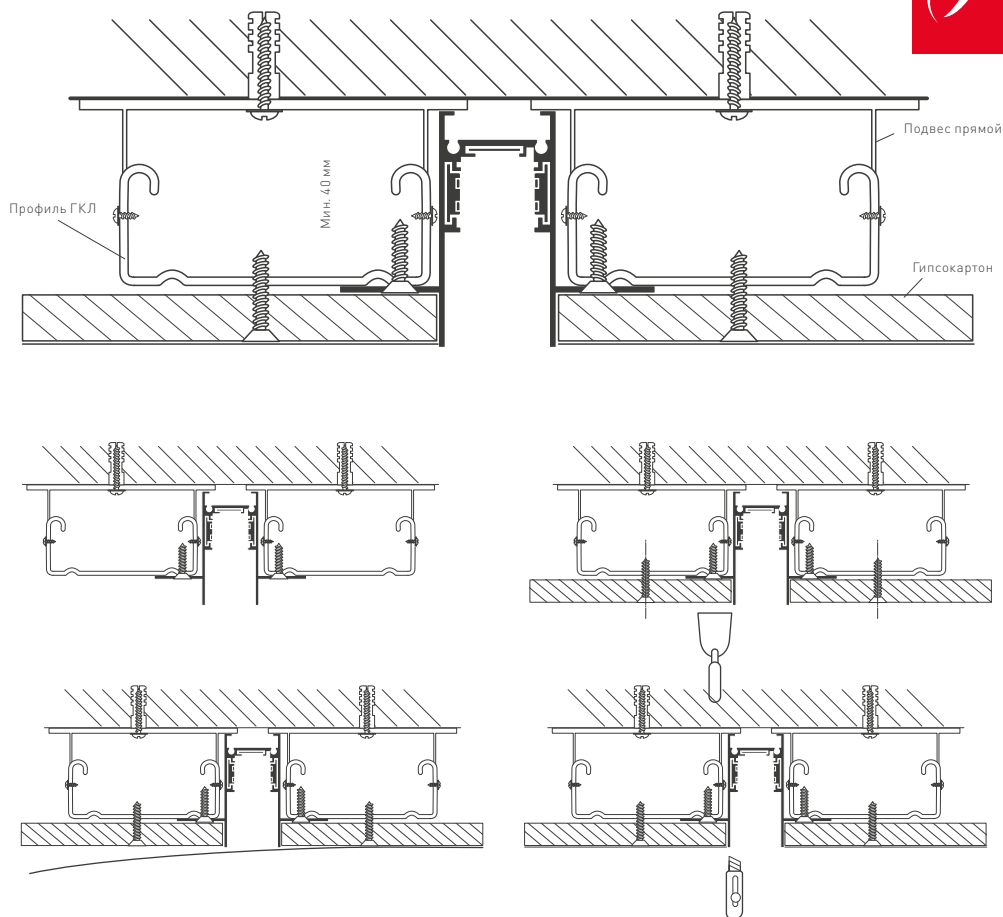
Рис. 3. Установка и подключение трека с одним слоем гипсокартона
